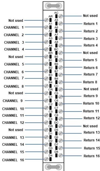
2591-A Wiring Diagram
